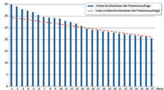
DURCHLAUFZEITEN DER ABGESCHLOSSENEN FERTIGUNGS-AUFTRÄGE
